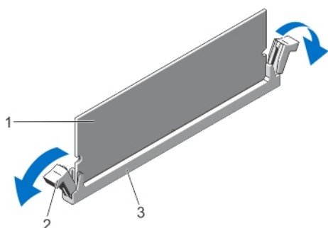
図 17. メモリモジュールの取り出し
