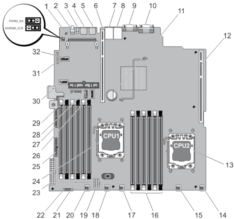
図 56. システム基板のコネクタとジャンパ
