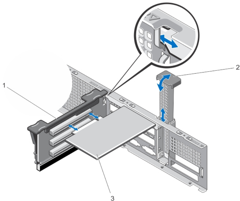
図 31. 拡張カードライザー 2 からの拡張カードの取り外しと取り付け
