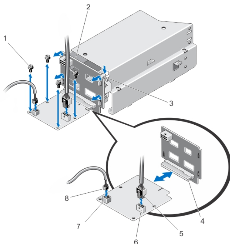
図 45. 配電基板の取り外しと取り付け
