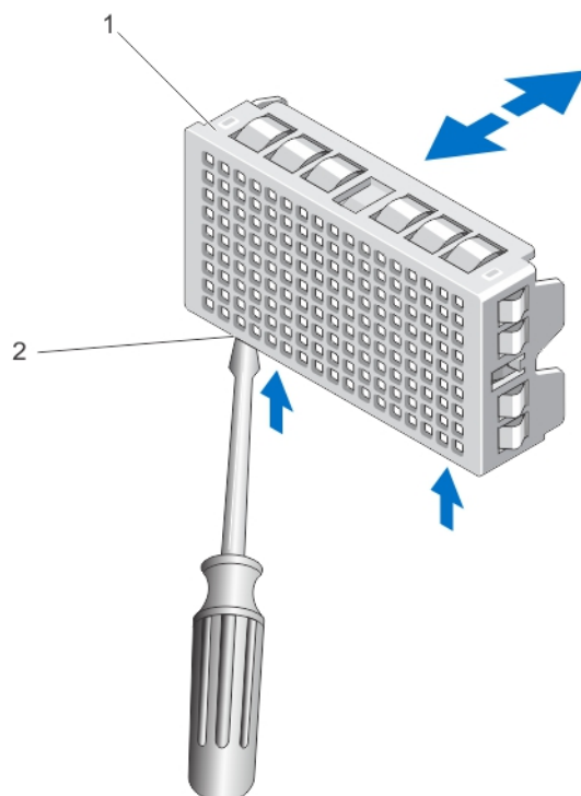
図 22.デュアルスロットハードドライブダミーの取り外しと取り付け
