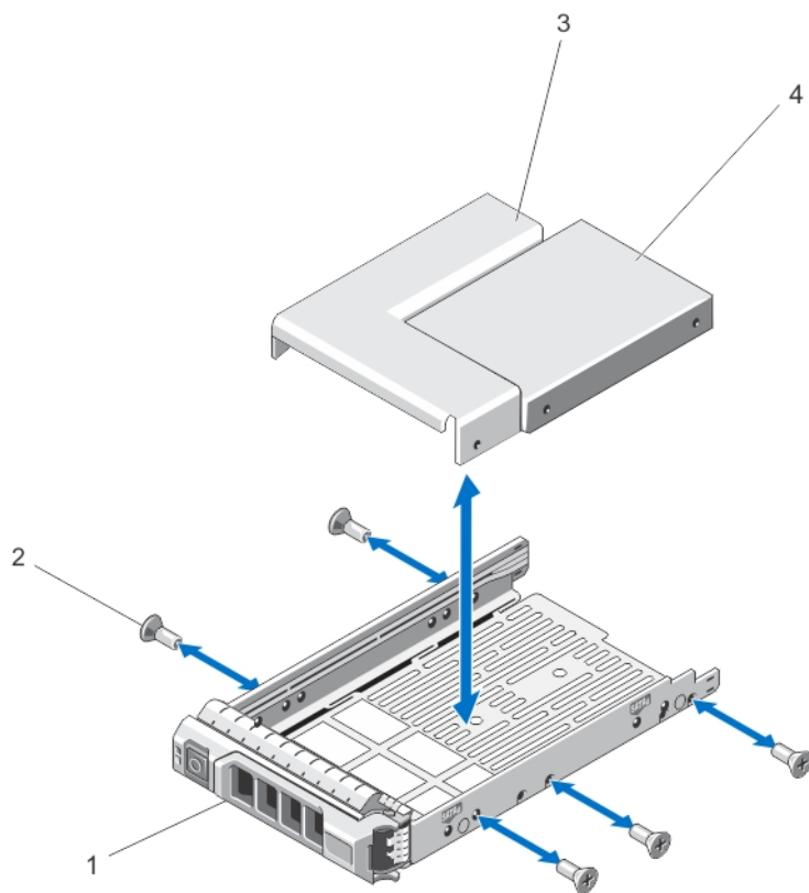
図 26. ハードドライブアダプタを 3.5 インチハードドライブキャリアから取り外す/取り付ける方法
