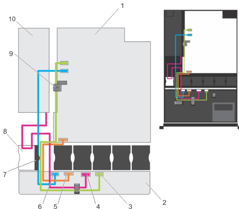
図 53. ケーブル接続図 — 非冗長電源ユニットシステムのハードドライブバックプレーン
