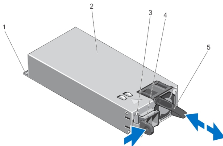
図 43. DC 電源装置の取り外しと取り付け
