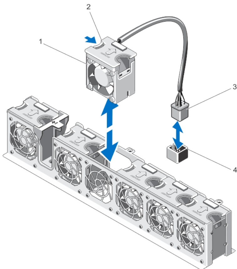
図 28. 冷却ファンの取り外しと取り付け
