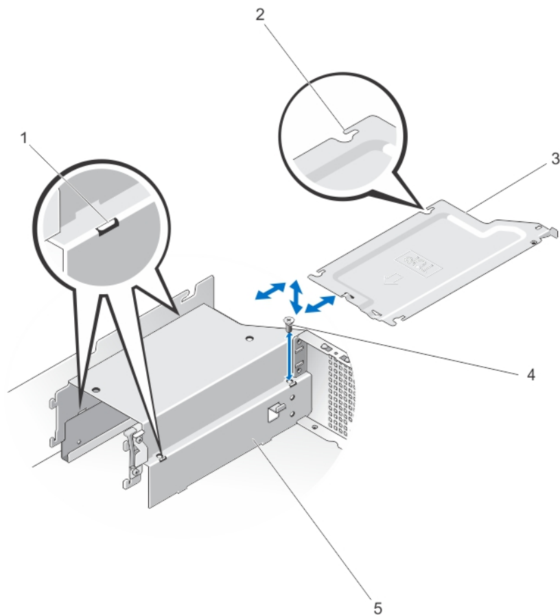
図 49. 冗長電源ユニット分岐器の取り外しと取り付け
