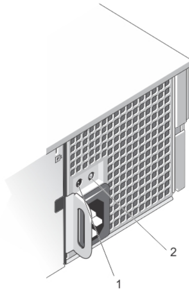
図 10. 非冗長 AC 電源装置のステータスインジケータと自己診断ボタン
