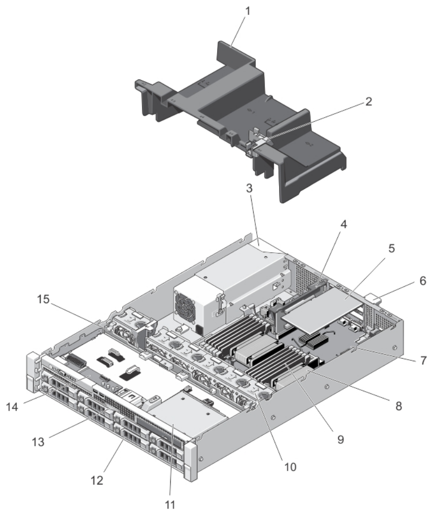
図 14. システムの内部 — 非冗長電源ユニットシャーシ
