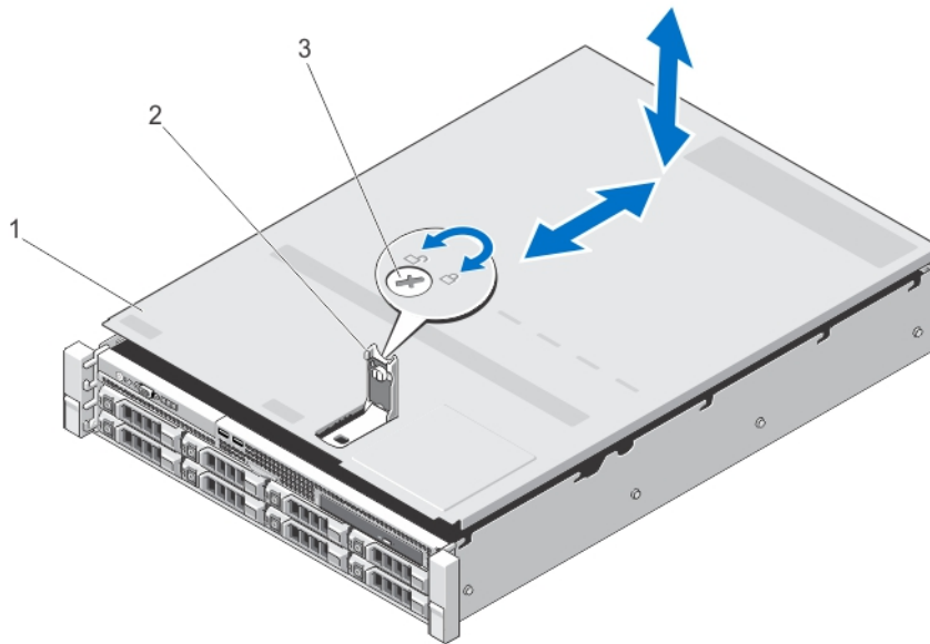
図 12. システムカバーの取り外しと取り付け
