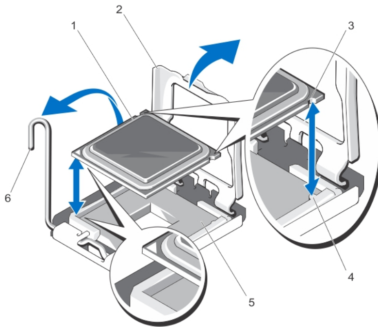
図 39. プロセッサの取り外しと取り付け
