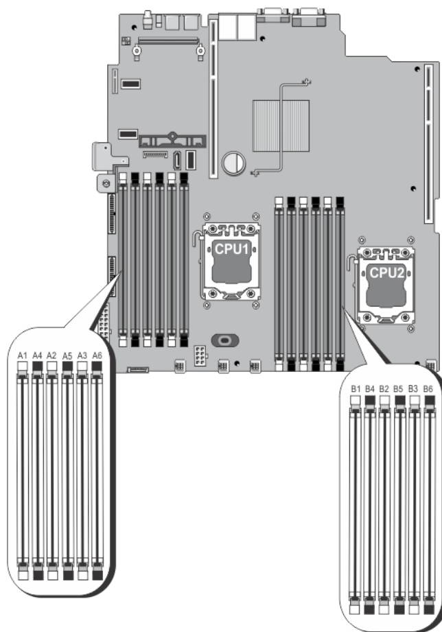
図 16. メモリソケットの位置
