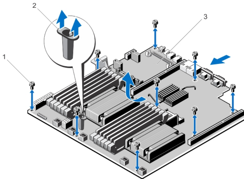
図 55. システム基板の取り外しと取り付け
