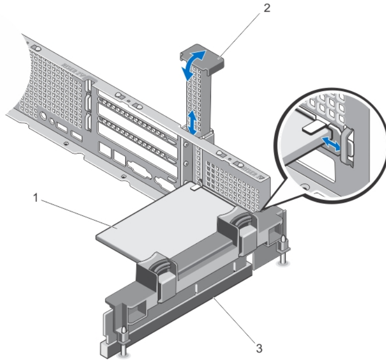
図 30. 拡張カードライザー 1 からの拡張カードの取り外しと取り付け
