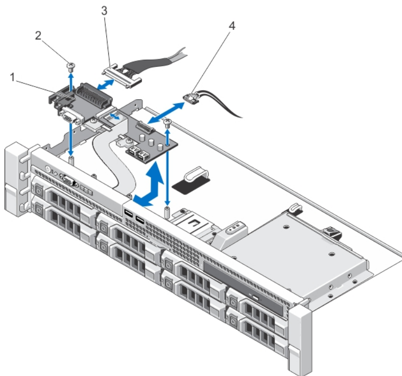
図 54. コントロールパネルボードの取り外しと取り付け
