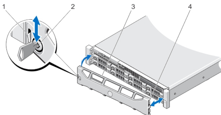
図 11. 前面ベゼルの取り付けと取り外し
