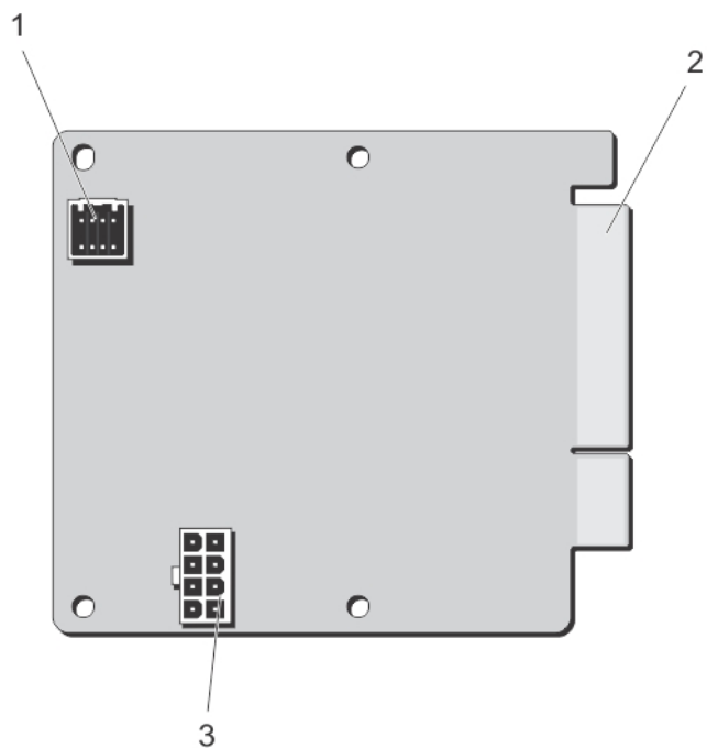
図 46. 配電基板コネクタ
