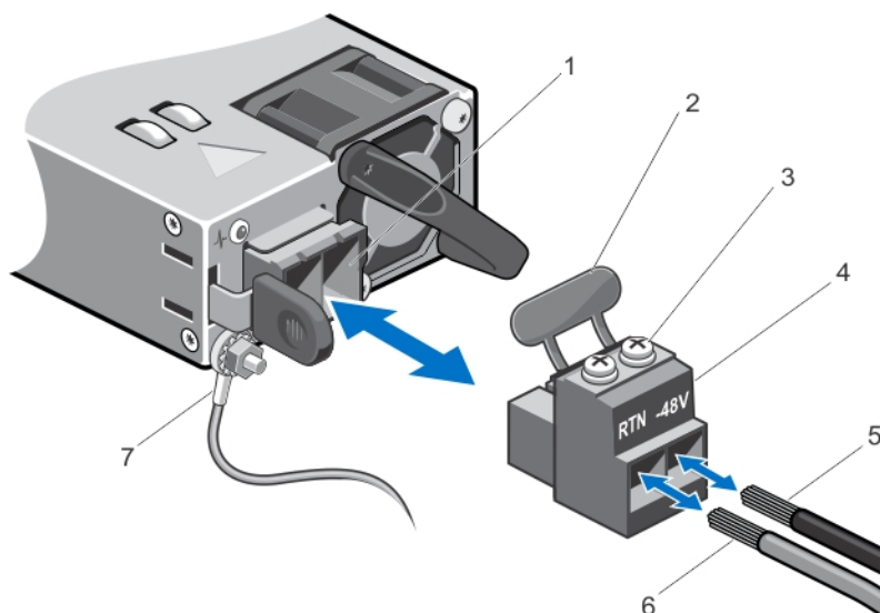
図 42. DC 入力電源ワイヤの編成
