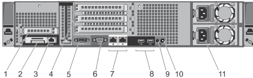
図 5. 背面パネルの機能とインジケータ — 冗長電源ユニットシャーシ
