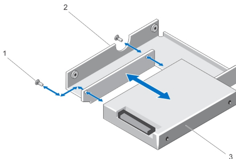
図 24. 2.5 インチハードドライブを 3.5 インチハードドライブアダプタから取り外す / 取り付ける方法
