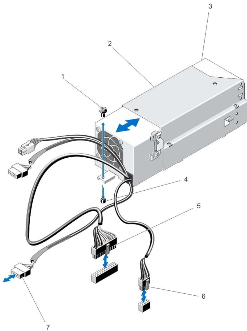
図 48. 非冗長電源ユニットの取り外しと取り付け
