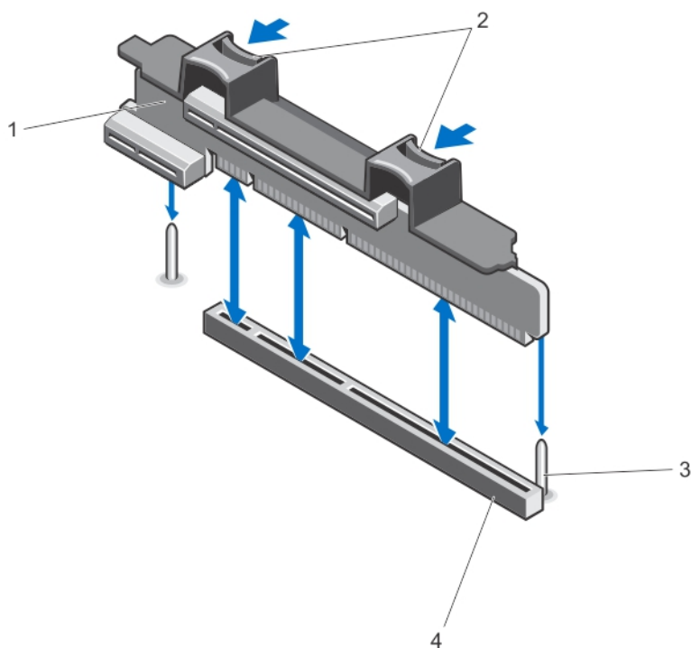
図 32. 拡張カードライザー 1 の取り外しと取り付け
