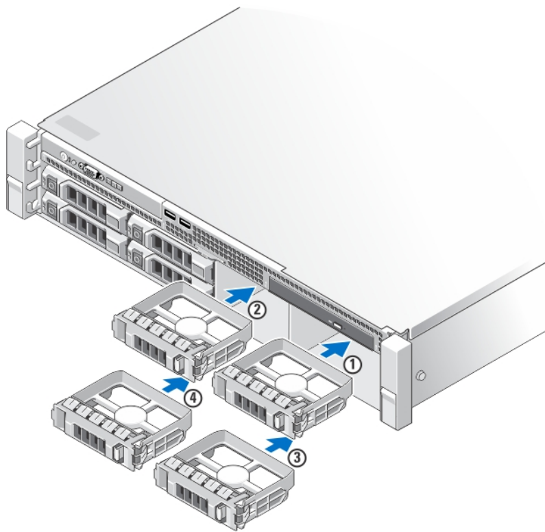
図 21. ハードドライブダミーの取り付け順序
