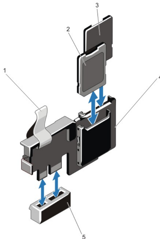
図 36. 内蔵デュアル SD モジュールの取り外しと取り付け
