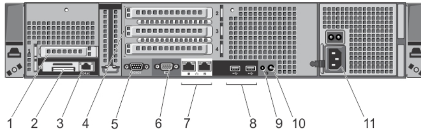
図 6. 背面パネルの機能とインジケータ — 非冗長電源ユニットシャーシ
