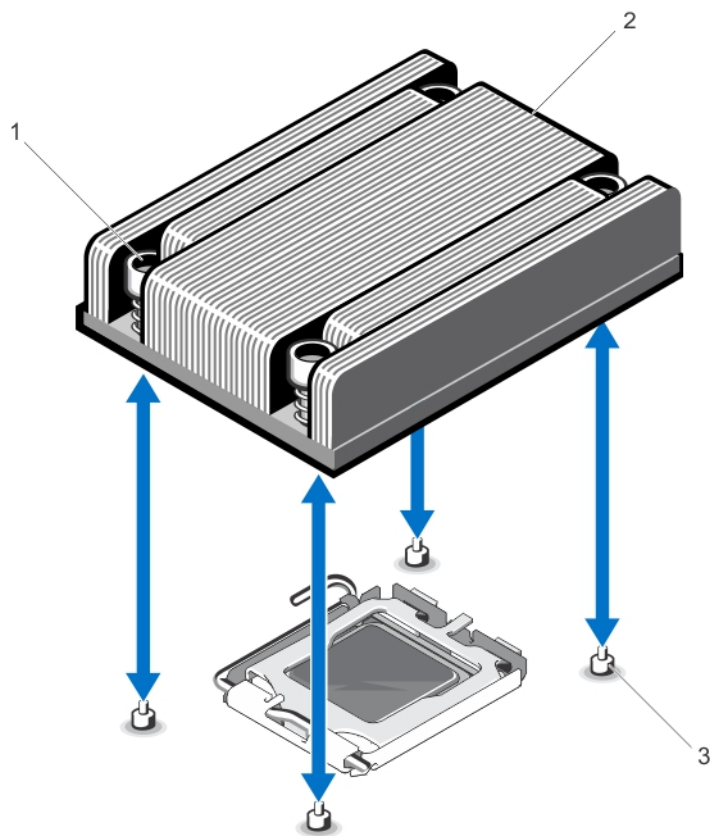
図 38. ヒートシンクの取り外しと取り付け
