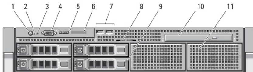
図 2. ソフトウェア RAID システムの前面パネルの機能とインジケータ
