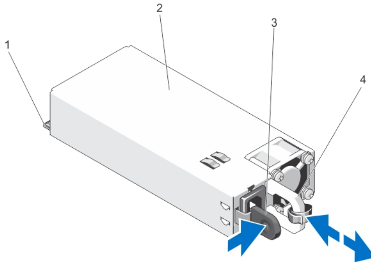
図 40. AC 電源装置の取り外しと取り付け
