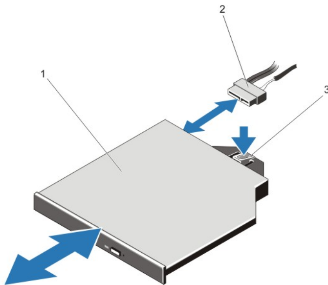
図 27. オプティカルドライブの取り外しと取り付け
