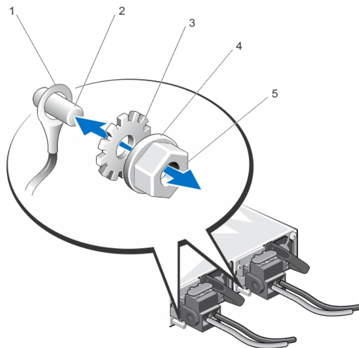
図 41. 保安接地線の編成と接続
