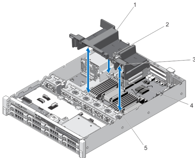
図 15. 冷却用エアフローカバーの取り外しと取り付け
