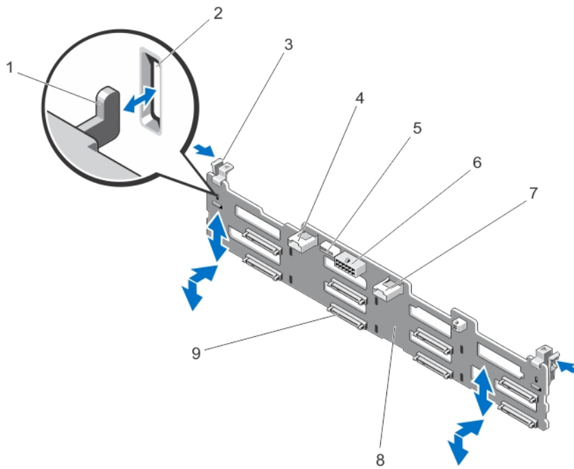
図 51. ハードドライブバックプレーンの取り外しと取り付け
